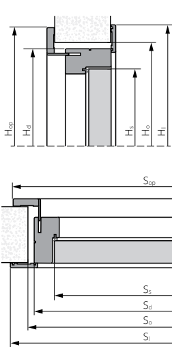
EI30 PLUS, EI60 PLUS NASTAVITELNÁ KOVOVÁ ZÁRUBEŇ
