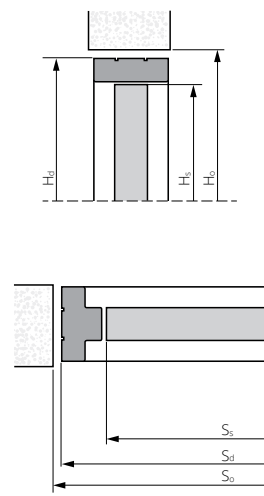
KYVNÉ DVEŘE PEVNÁ DŘEVĚNÁ ZÁRUBEŇ
