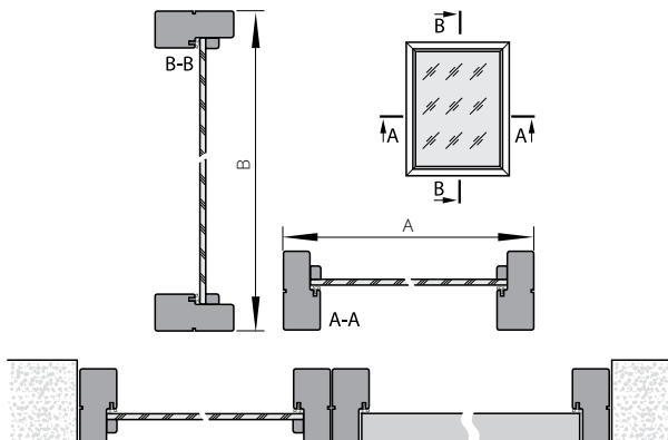
BEZFALCOVÝ SYSTÉM
