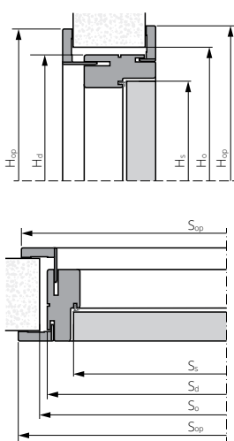
ZVUKOVĚ IZOLAČNÍ TYP A, B BEZPOLODRAŽKOVÁ DŘEVĚNÁ ZÁRUBEŇ
