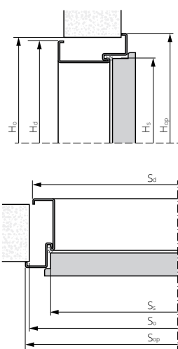
EI30 PLUS, EI60 PLUS, RC3, GAMMA, DECO INVEST, CERBER PLUS PEVNÁ KOVOVÁ ZÁRUBEŇ
