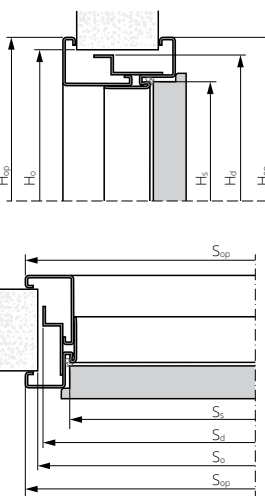
ZVUKOVĚ IZOLAČNÍ TYP A, B, DECO INVEST, GAMMA NASTAVITELNÁ KOVOVÁ ZÁRUBEŇ
