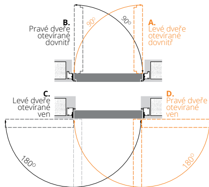
JEDNOKŘÍDLÉ DVEŘE
