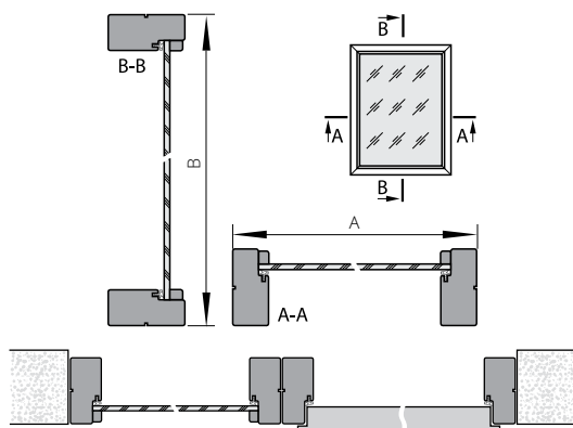
FALCOVÝ SYSTÉM
