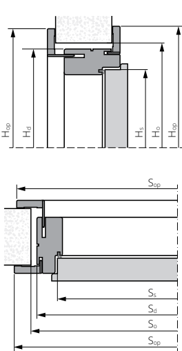
FR EI30 (OBOUSTRANNÁ REGULACE) ZVUKOVĚ IZOLAČNÍ TYP A, B DŘEVĚNÁ ZÁRUBEŇ
