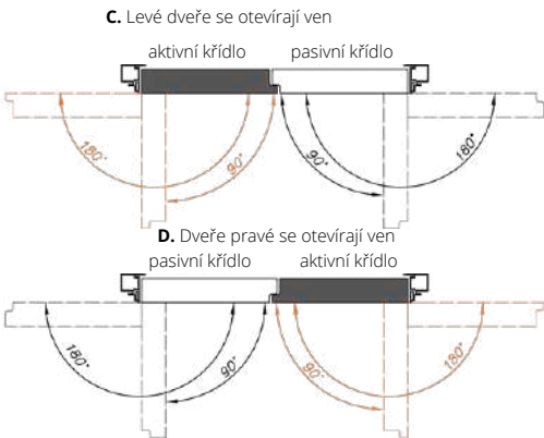
DVOUKŘÍDLÉ DVEŘE
