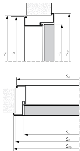
EI30 PLUS, EI60 PLUS, HIGRO PEVNÁ KOVOVÁ ZÁRUBEŇ
