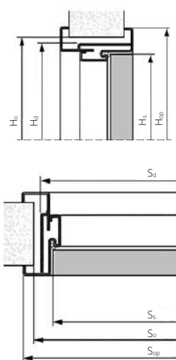
EI30 PLUS, EI60 PLUS NASTAVITELNÁ KOVOVÁ ZÁRUBEŇ
