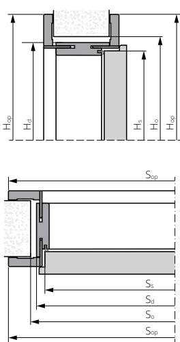
ZVUKOVĚ IZOLAČNÍ TYP A, B NASTAVITELNÁ ZÁRUBEŇ DIN ZP
