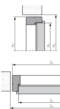
ZVUKOVĚ IZOLAČNÍ TYP A, B PEVNÁ DŘEVĚNÁ ZÁRUBEŇ
