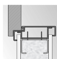
záruběň Rohová VELKÁ montáž na stěně SDK
