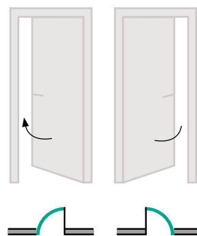
DVEŘE S REVERZNÍ POLODRÁŽKOU LEVÉ KŘÍDLO PRAVÉ KŘÍDLO
