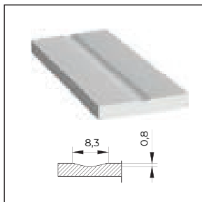
detail frézování
