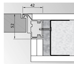
Reverzní polodrážka (otevírané dovnitř)
