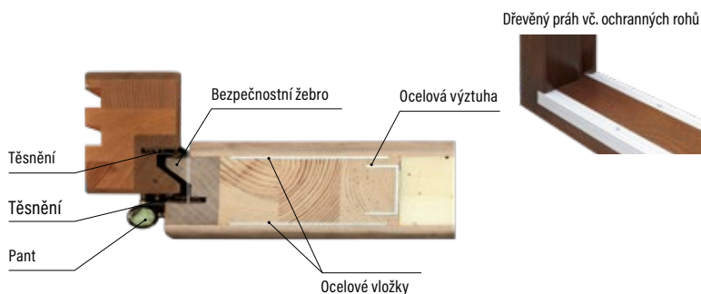
Dřevěný práh vč. ochranných rohů
